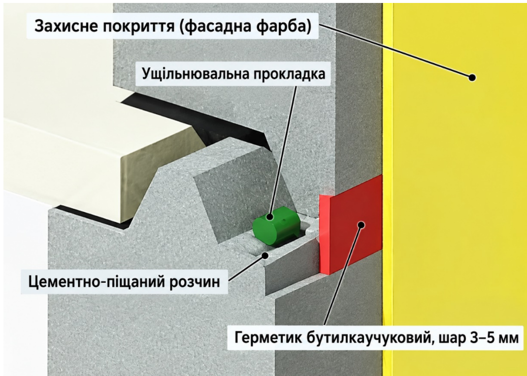
Мал.3 Влаштування горизонтального стику.
