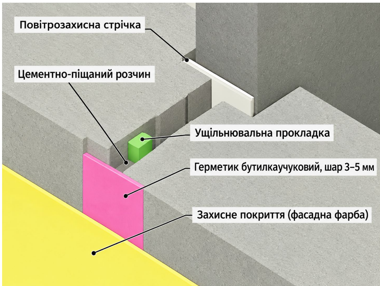
Мал.1 Герметизація стику зовнішніх панелей.
